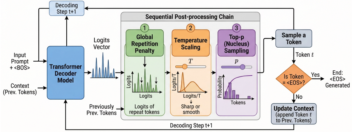
Figure 3 확률적 샘플링과 페널티 메커니즘 도입
