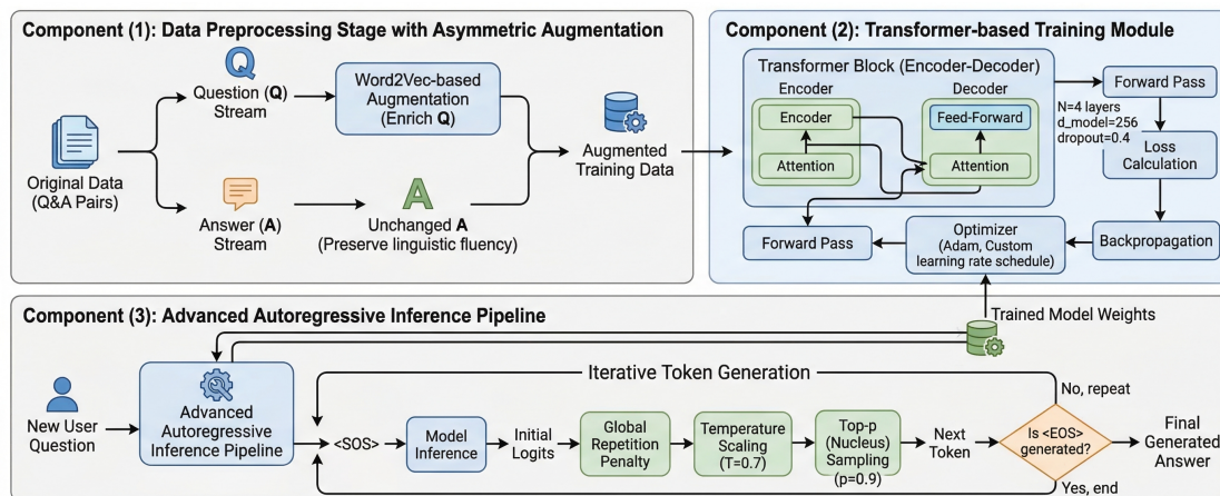
Figure 1 전체 시스템 아키텍처
